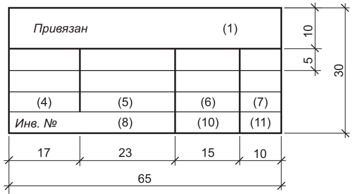
Рисунок Н.2 — Штамп привязки (последующие листы документа)
