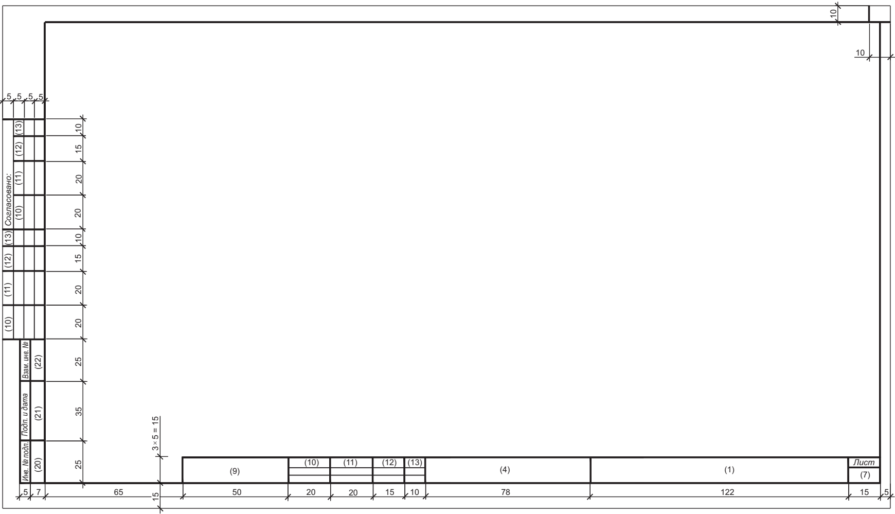
Рисунок Е.5 — Допустимая форма основной надписи, дополнительных граф к ней для последующих листов основных комплектов чертежей, чертежей разделов проектной документации
